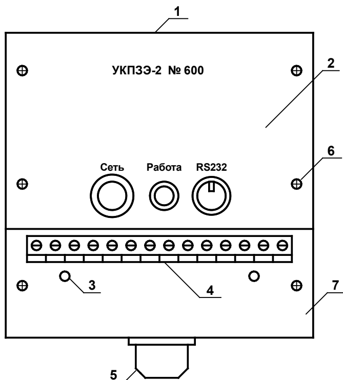
Рисунок 5.1. Общий вид УКПЗЭ: 1 – корпус; 2 – верхняя крышка; 3 – крепежное отверстие; 4 – клемная колодка; 5- кабельный зажим; 6 – крепежные шурупы крышек; 7 – нижняя крышка.
