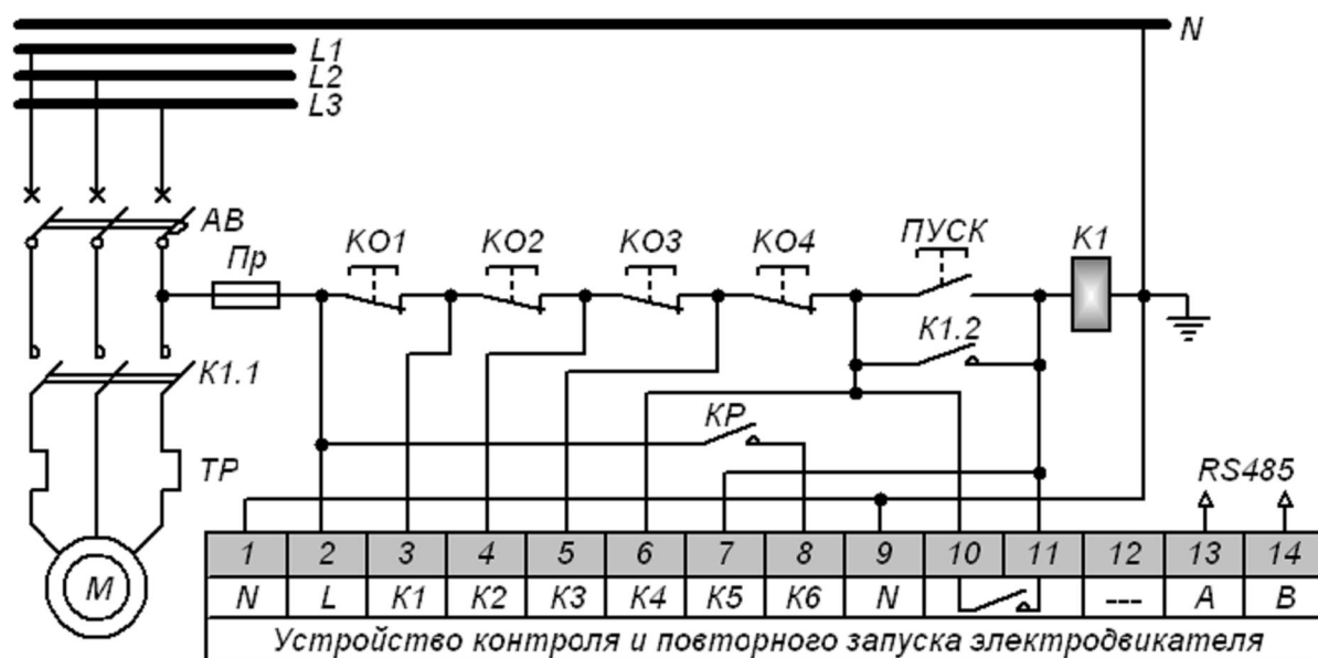
Рисунок 7.1. Схема электрическая соединений УКПЗЭ.
